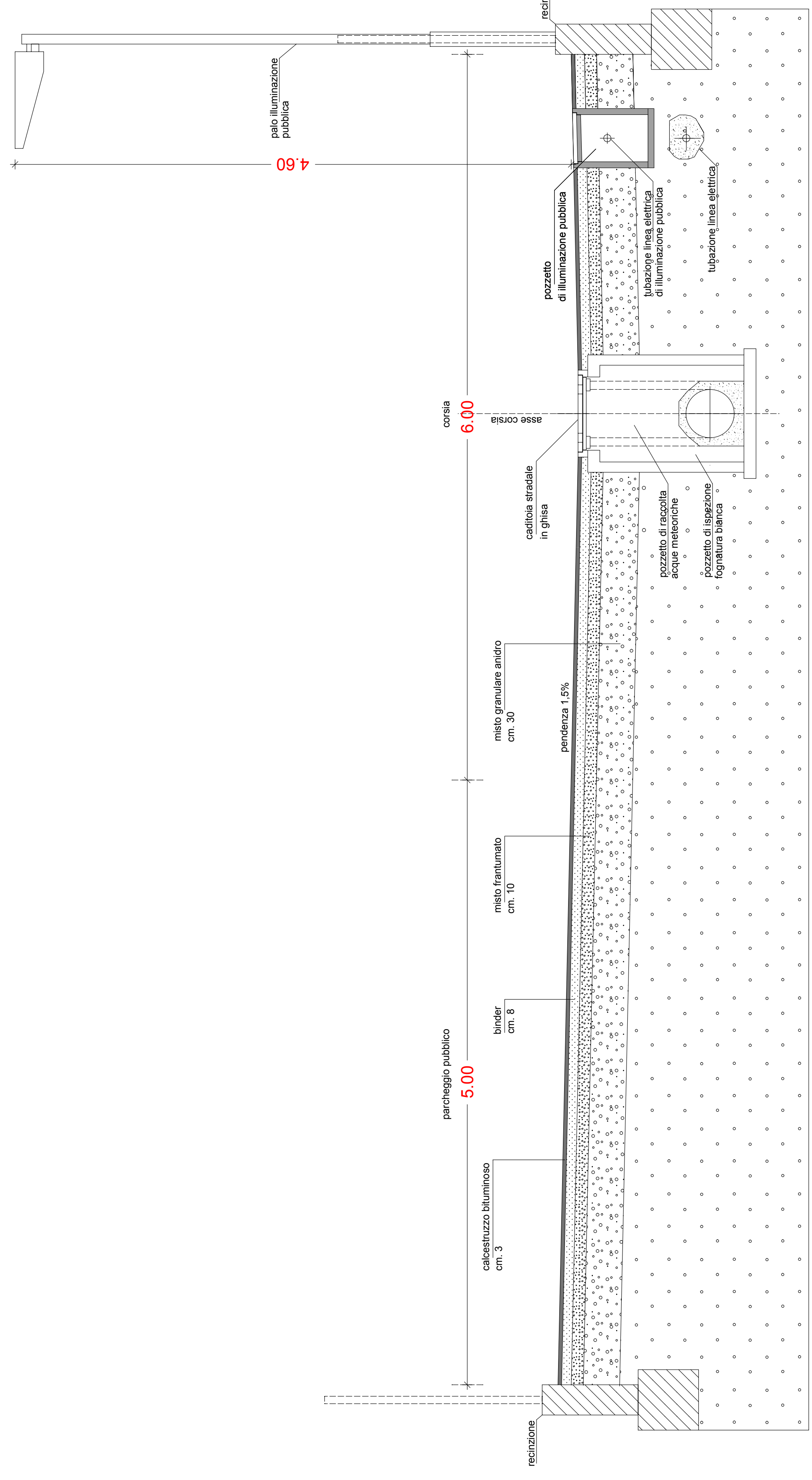
Sezione O.O.U.U. su parcheggio pubblico Scala 1/25
